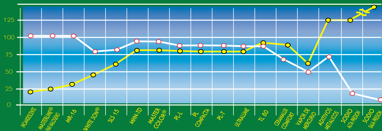
RELACION ENTRE EL ÍNDICE DE RENDIMIENTO DE COLOR (CRI) Y LA EFICIENCIA DE ALGUNAS LAMPARAS PHILIPS
