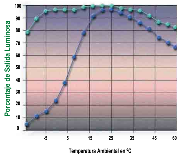
Flujo Luminoso en Lúmenes vs. Temperatura Ambiental
